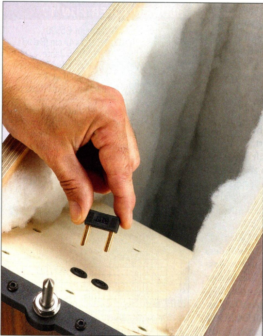
Die Impedanzlinearisierung soll empfindlicheren Röhrenverstärkern die Zusammenarbeit erleichtern und ist im Horn am Boden der Fun 17 steckbar
